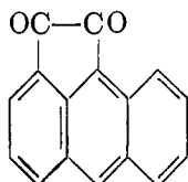
VI Aceanthraquinone
